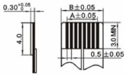
适用扁平电缆 Proper cable
