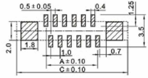
反针 PCB 寸法 Versa needle PCB LAYOUT
