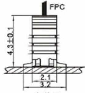
安装图 ASSEMBLY LAYOUT
