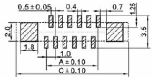
正针 PCB 寸法 Positive needle PCB LAYOUT
